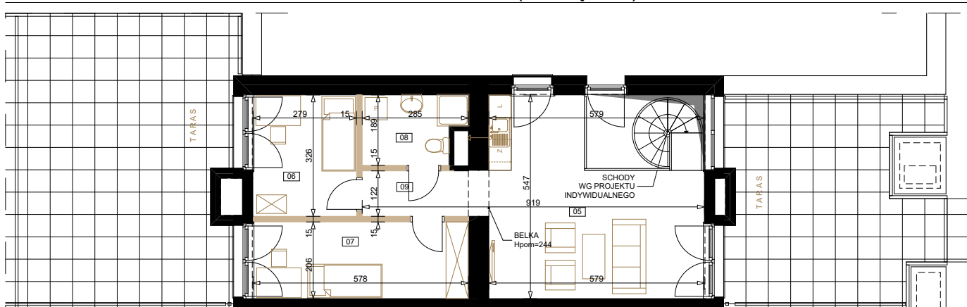
C/75 - POZIOM 2 (VI PIĘTRO)
